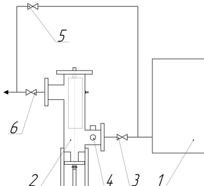
Рисунок 2 – Схема обвязки установки ЩИТ-4Н: 1 – подогреватель воды; 2 – устройство растворения анода; 3 – входная задвижка; 4 – датчик скорости потока; 5 – байпасная задвижка; 6 – исходная задвижка.
