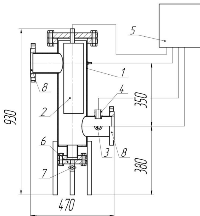
Рисунок 1 – Схема установки ЩИТ-4Н: 1 – прибор растворения анода; 2 – анод А-2; 3 – датчик скорости потока ДП-2; 4 – датчик скорости коррозии ДК-1; 5 – электронный блок БЭЩ-2Н; 6 – крышка люка; 7 – шаровой кран; 8 – фланцы D_f=100 , P_f = 1,6 МПа.
