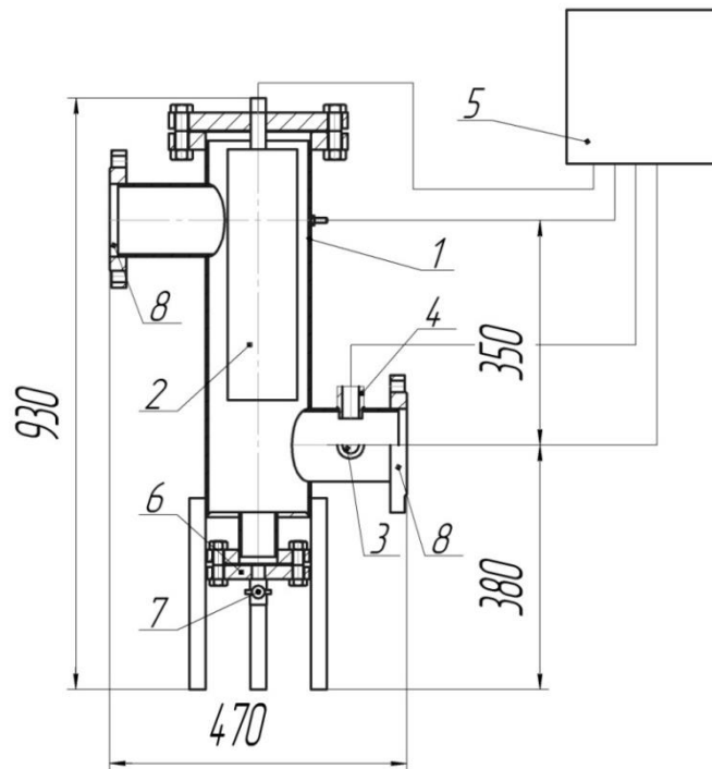
Рисунок 1 – Схема установки ЩИТ-4Н: 1 – пристрій розчинення анода; 2 – анод А-2; 3 – датчик швидкості потоку ДП-2; 4 – датчик швидкості корозії ДК-1; 5 – електронний блок БЕЩ-2Н; 6 – кришка люка; 7 – шаровий кран; 8 – фланці D_y=100 , P_y = 1,6 МПа.
