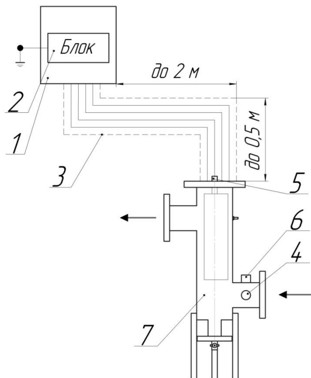
Рисунок 3 – Схема електричного монтажу установки ЩИТ-4Н: 1 – шафа захисна, 2 – блок електронний БЕЩ-4Н, 3 – закритий короб, 4 – датчик швидкості потоку, 5 – контактор анода, 6 – датчик швидкості корозії, 7 – пристрій розчинення анода.
