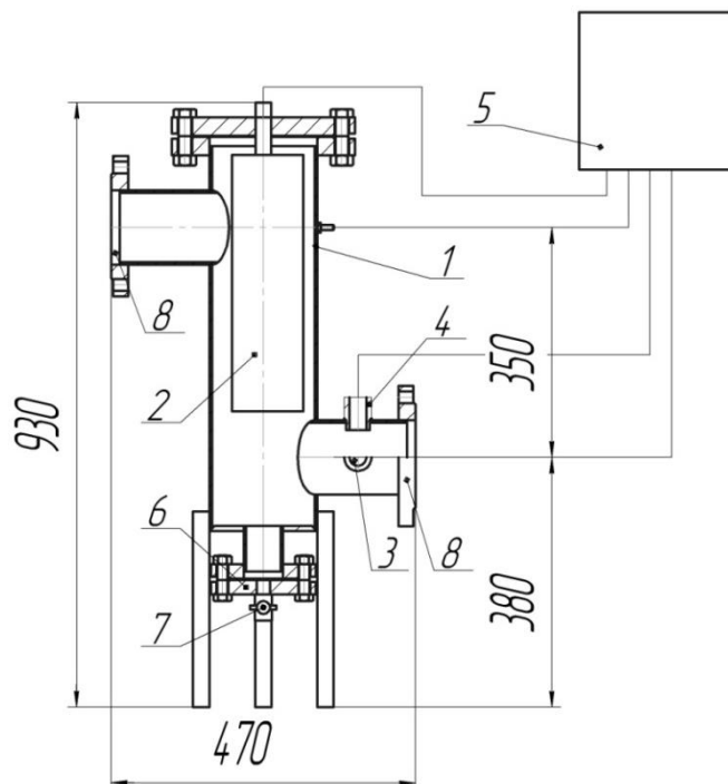
Рисунок 1 – Схема установки ЩИТ-2Н: 1 – пристрій розчинення анода; 2 – анод А-2; 3 – датчик швидкості потоку ДП-2; 4 – датчик швидкості корозії ДК-1; 5 – електронний блок БЕЩ-2Н; 6 – кришка люка; 7 – шаровий кран; 8 – фланці D_y=100 , P_y = 1,6 МПа.
