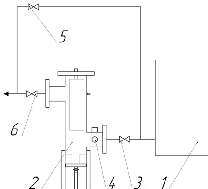
Рисунок 2 – Схема обв'язки установки ЩИТ-2Н: 1 – підігрівач води; 2 – пристрій розчинення анода; 3 – вхідна засувка; 4 – датчик швидкості потоку; 5 – байпасна засувка; 6 – вихідна засувка.
